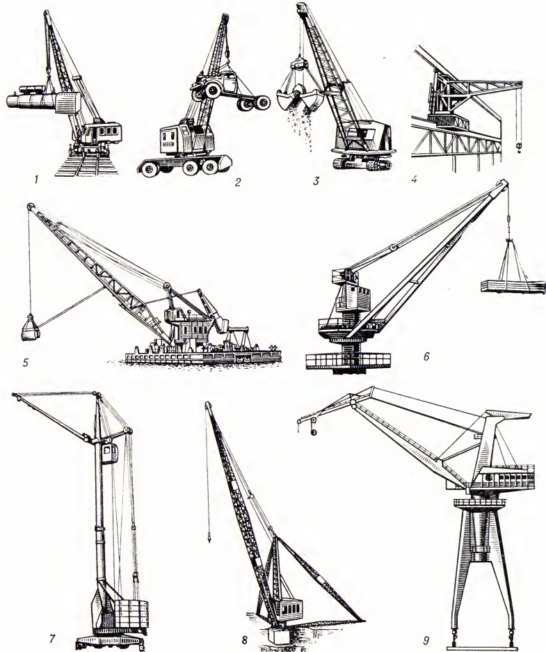
Рис. 1. Поворотные краны: 1 — железнодорожный; 2 — пневмоколёсный; 3 — гусеничный; 4 — настенно-поворотный передвижной; 5 — плавучий; 6 — судовой; 7 — башенный; 8 — мачтово-стреловой; 9 — порталный.
